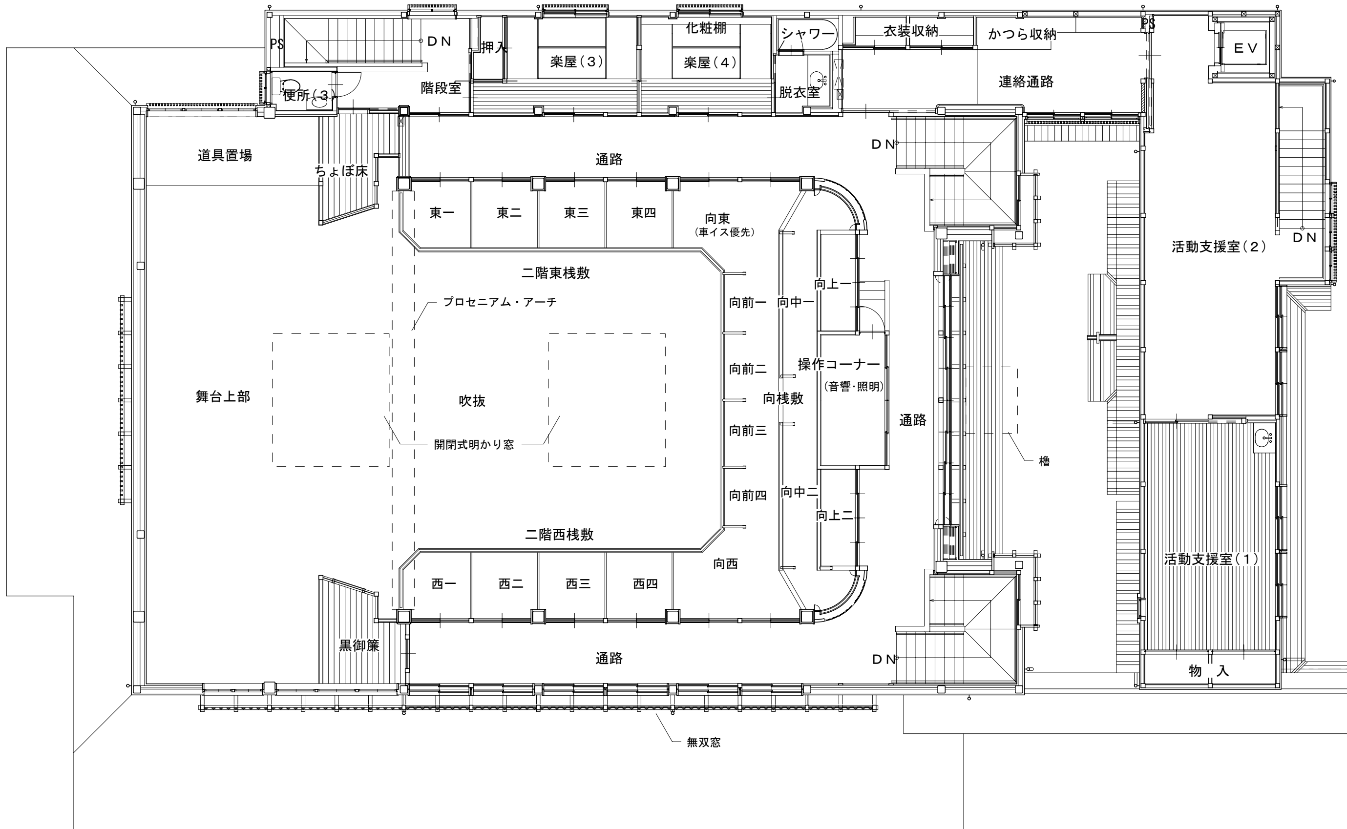
弁天座 2階平面図
